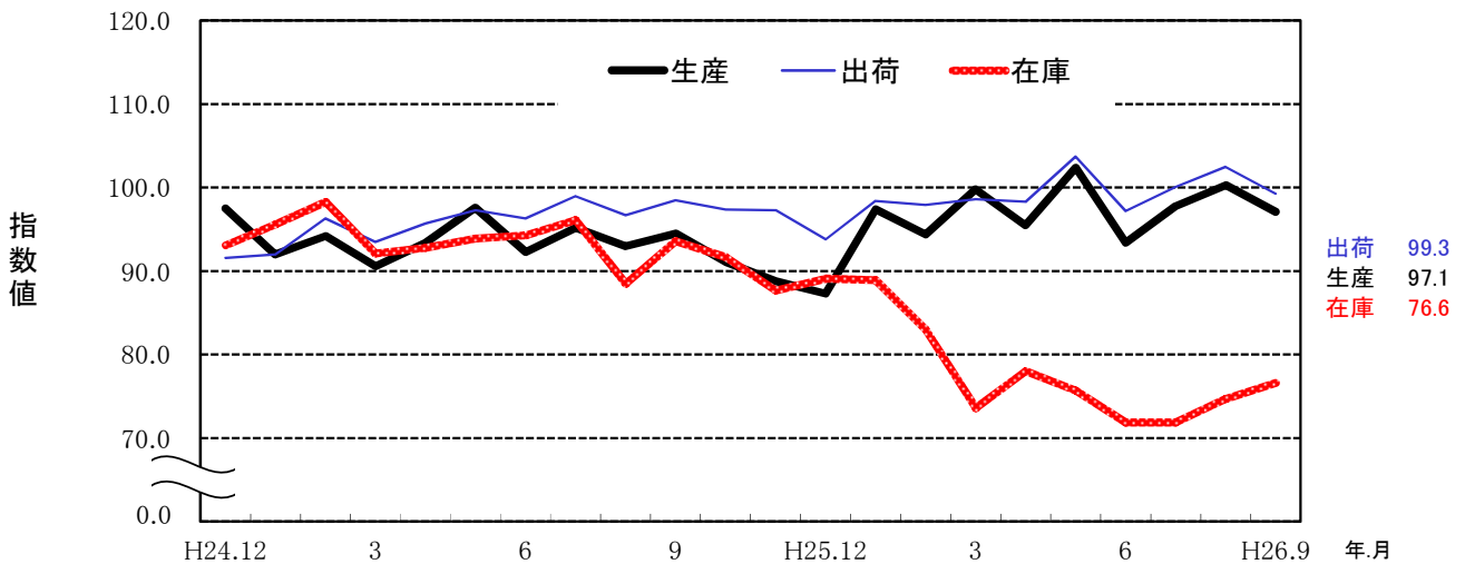
佐賀県鉱工業指数(季節調整済)の推移
