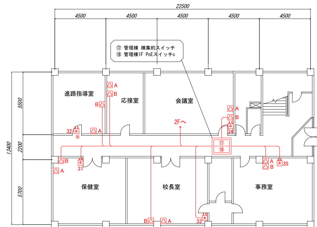
管理棟 1 F 平面図
