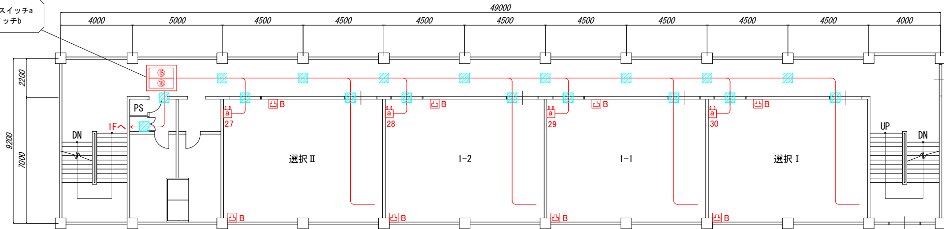
普通教室棟 3 F 平面図
