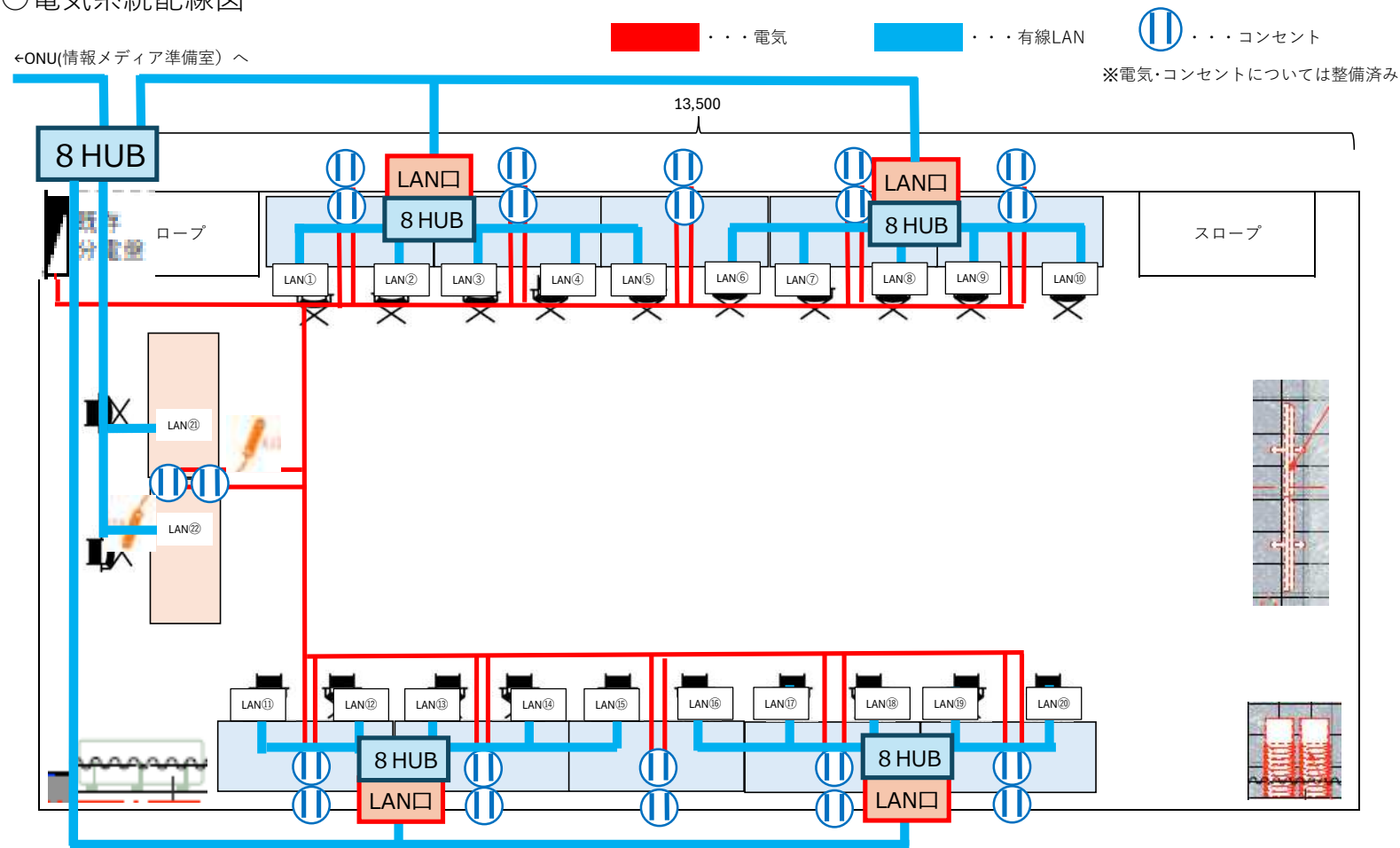
○電気系統配線図
