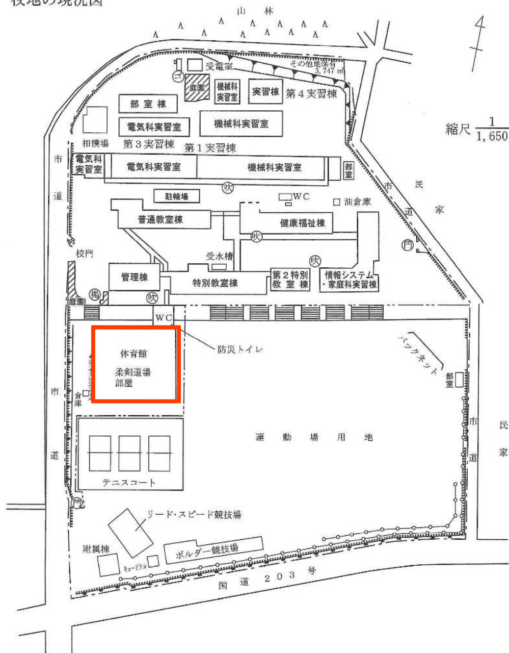
7-1) 校地の現況図
