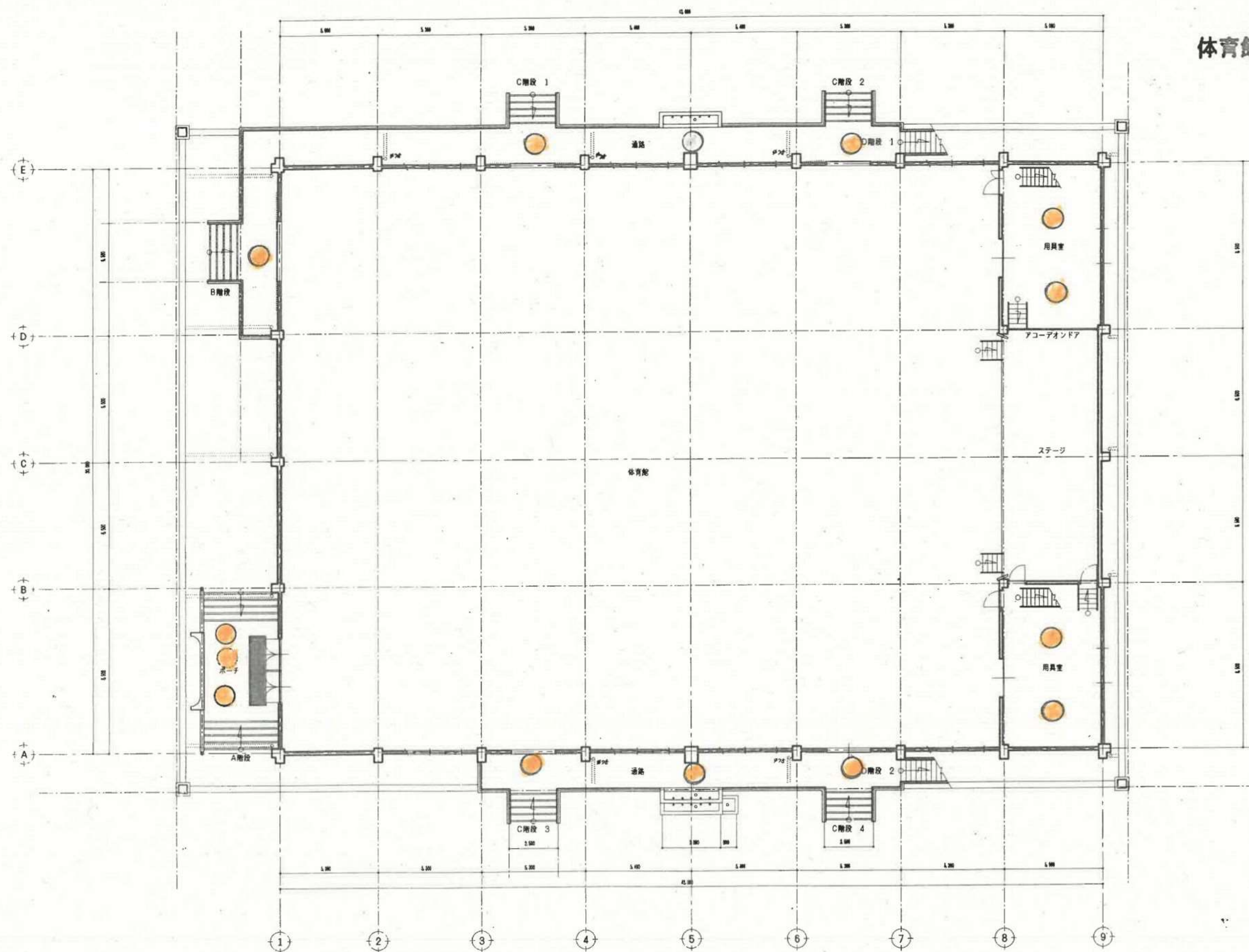
1階平面図
