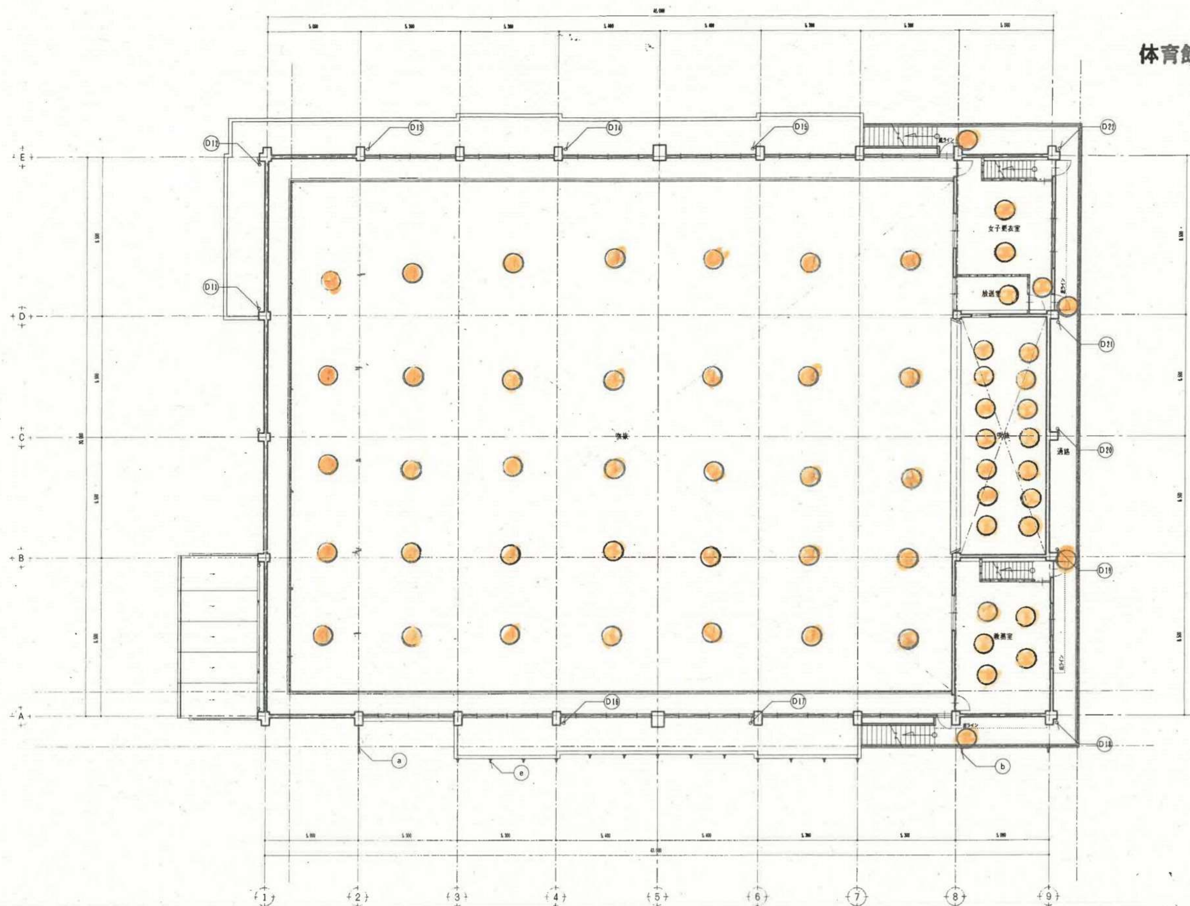
2階平面図
