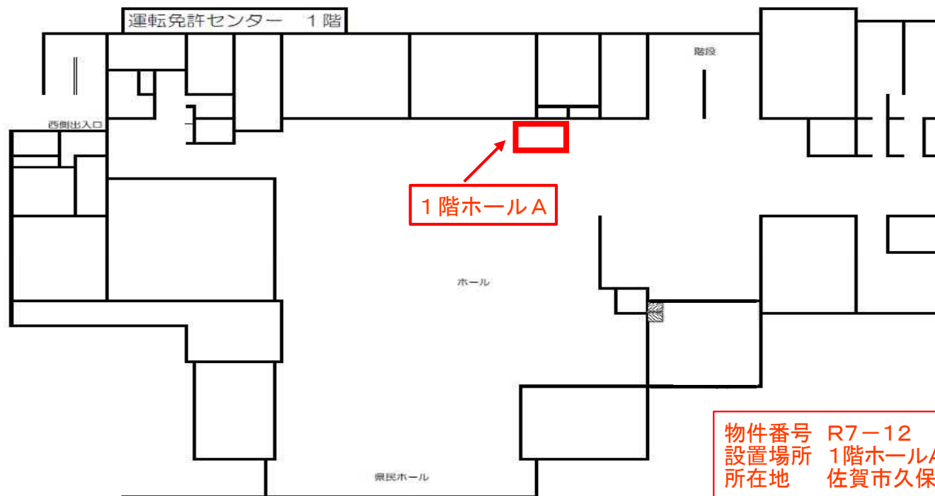
平面図
