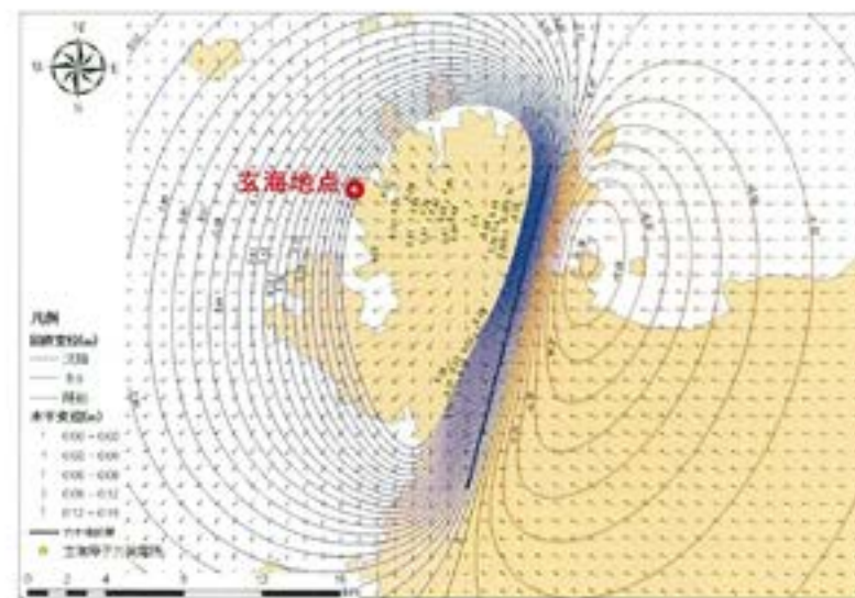
竹木場断層
