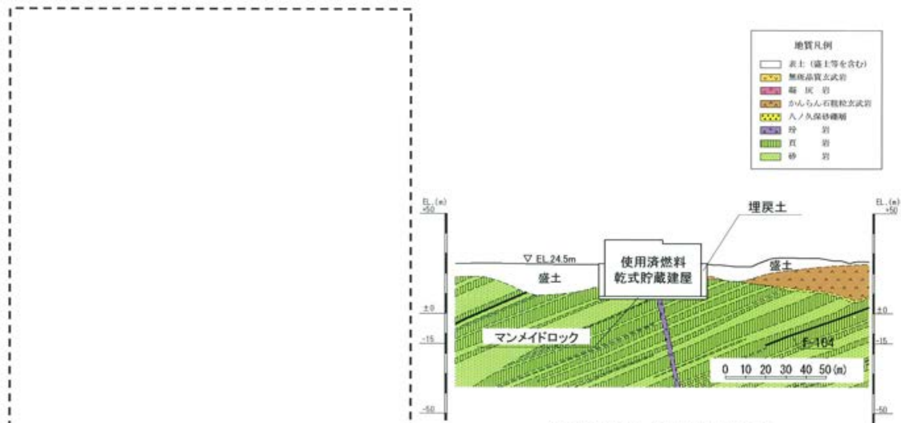
使用済燃料乾式貯蔵建屋断面図
