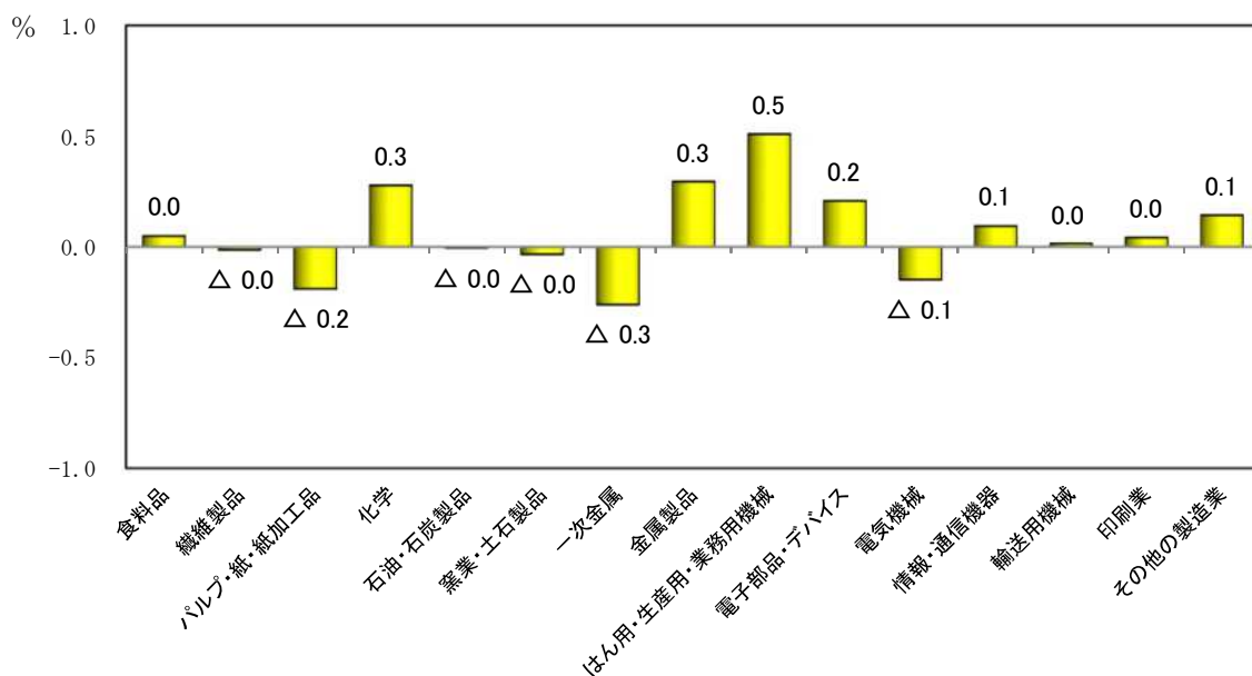
図10 製造業の業種別増加寄与度(令和3年度)
