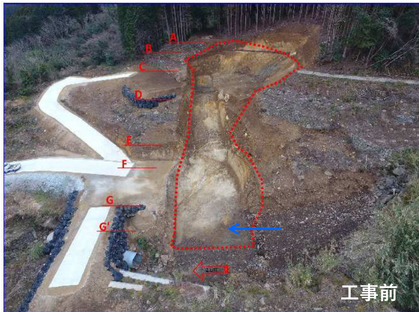
鳴石川砂防（整備状況）
