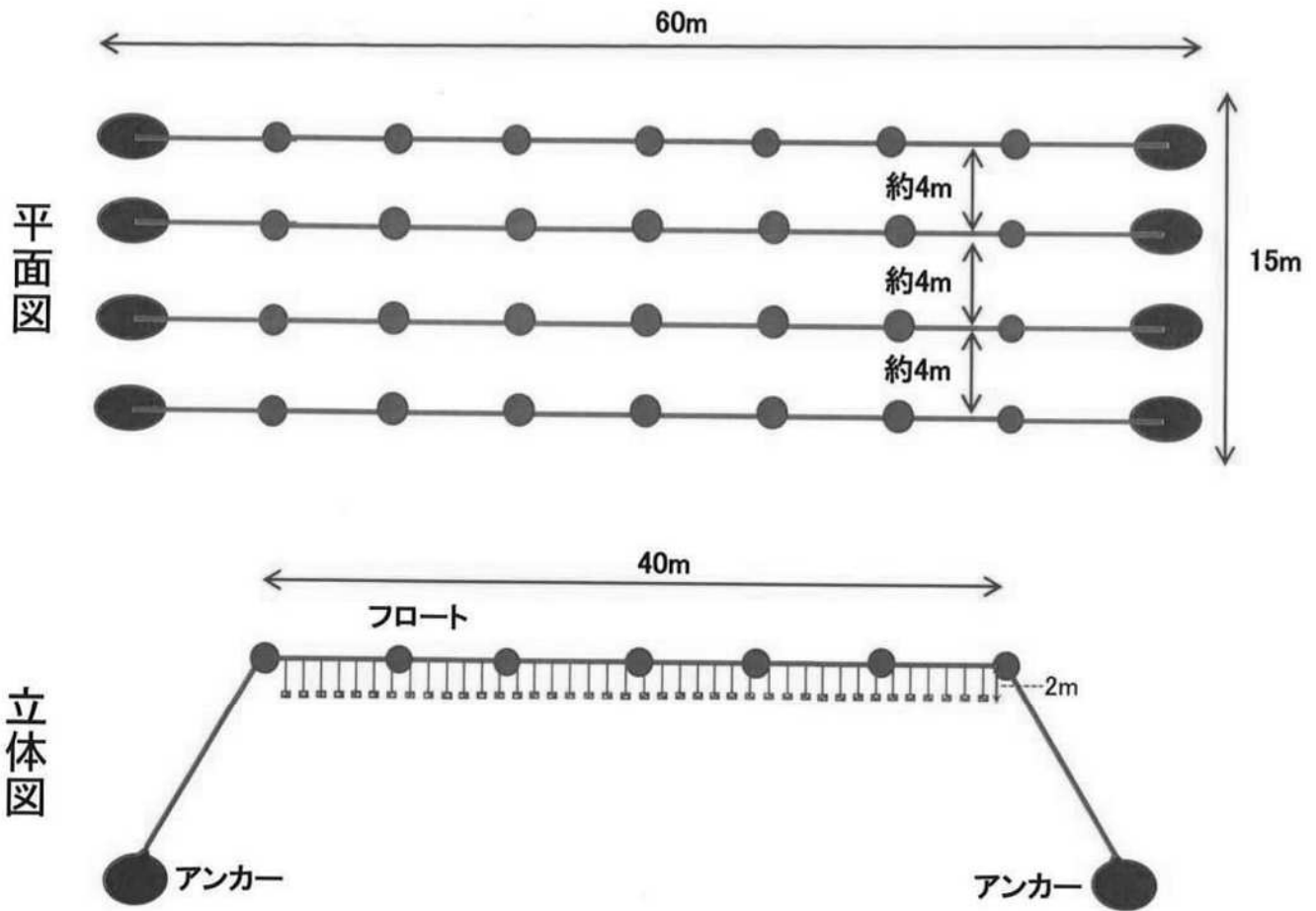
養殖施設概要図
