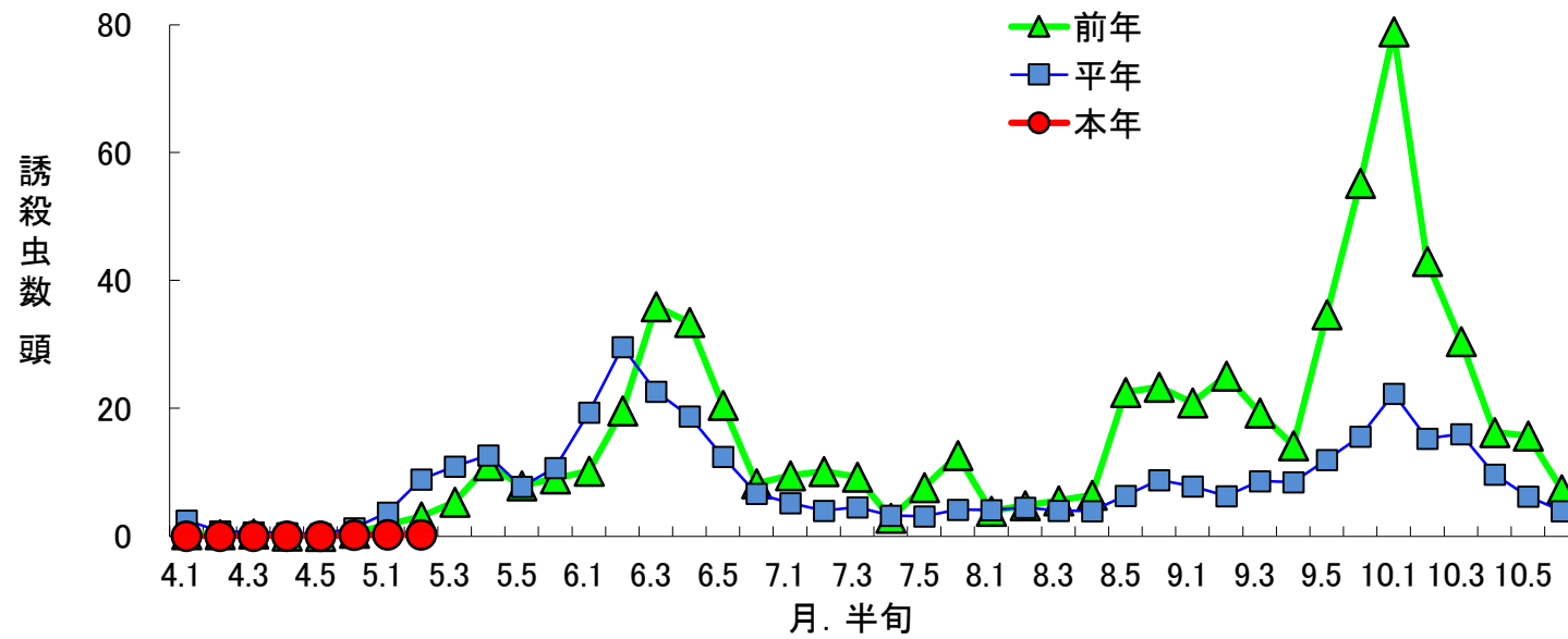
黄色粘着トラップによるチャノキイロアザミウマの誘殺数の推移(小城市 果樹試験場調査)
