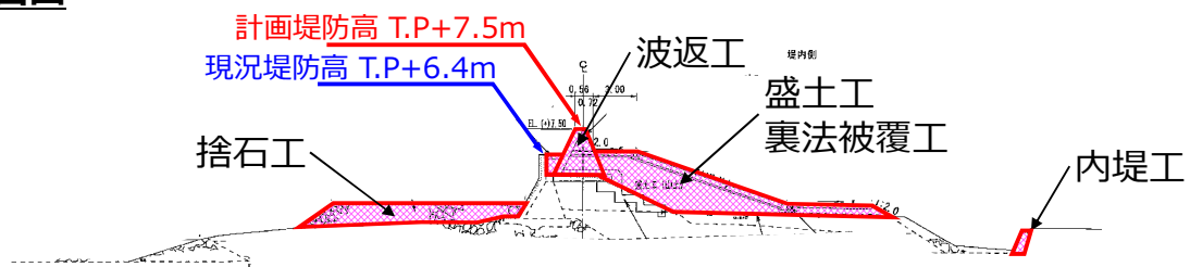
堤防断面図
