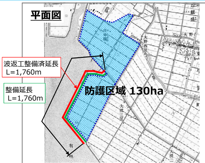
▲堤防の整備状況
