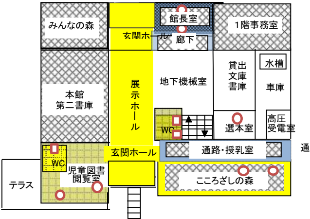
一階平面図
