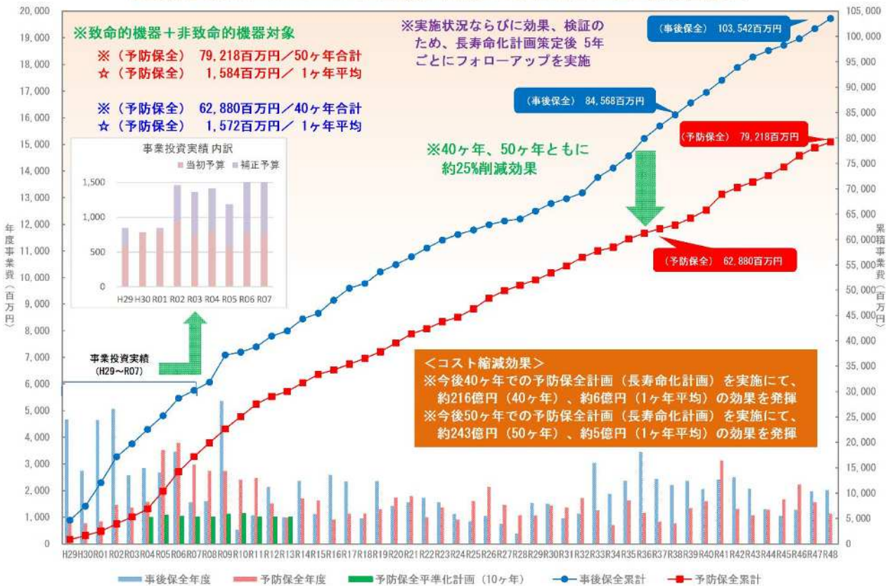
長期保全計画シミュレーション結果 (特構+対応+県単/全95施設対象)
