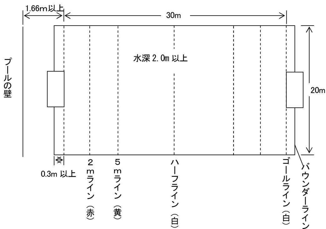
【別図 2】水球用プール
