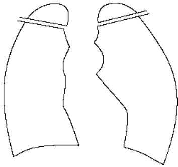
心胸比
