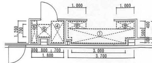
廃棄物等の保管施設詳細図 S=1/100
