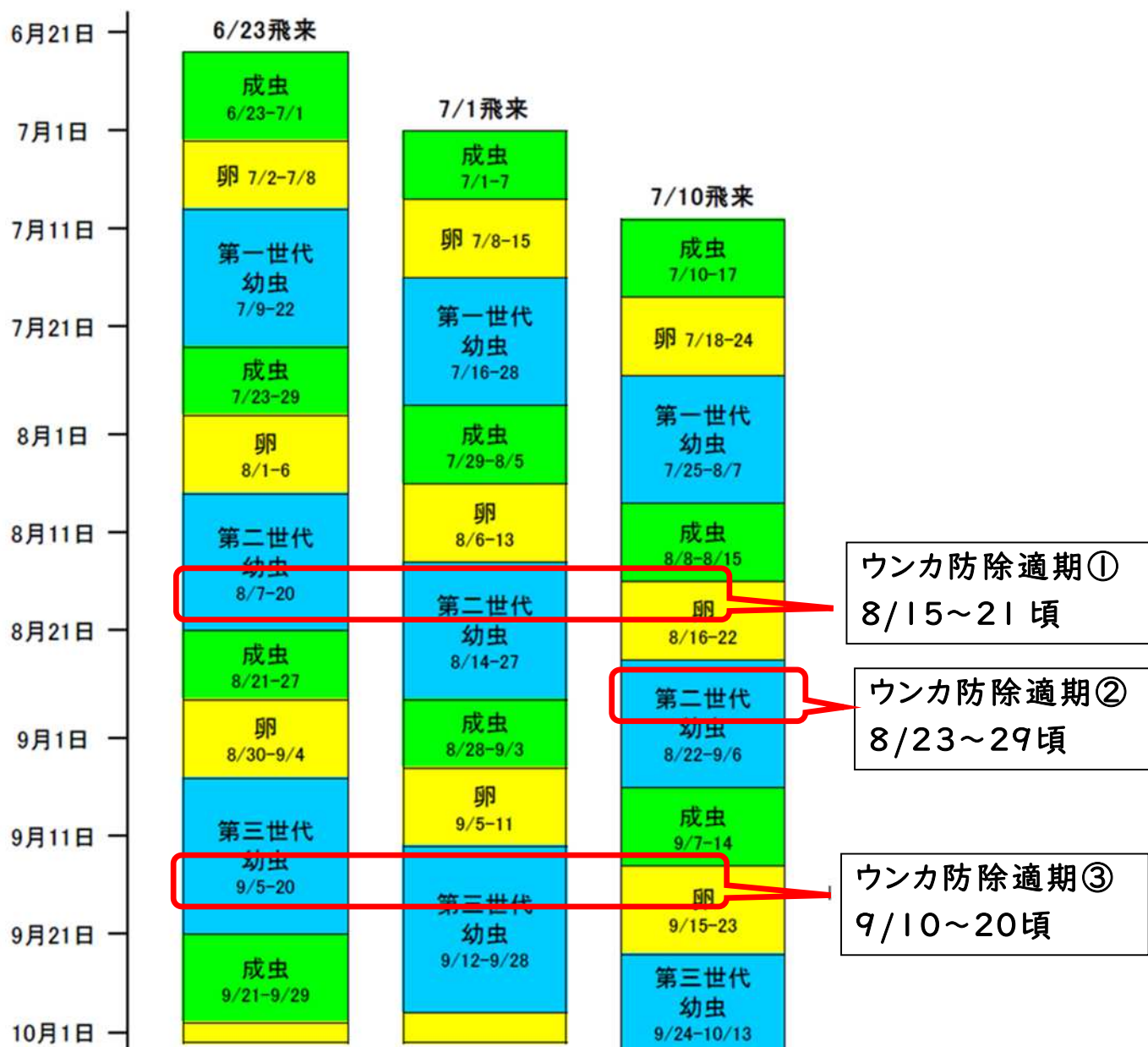
図1 トビイロウンカ各世代の発生予測（第2版、2024年7月19日作成）
