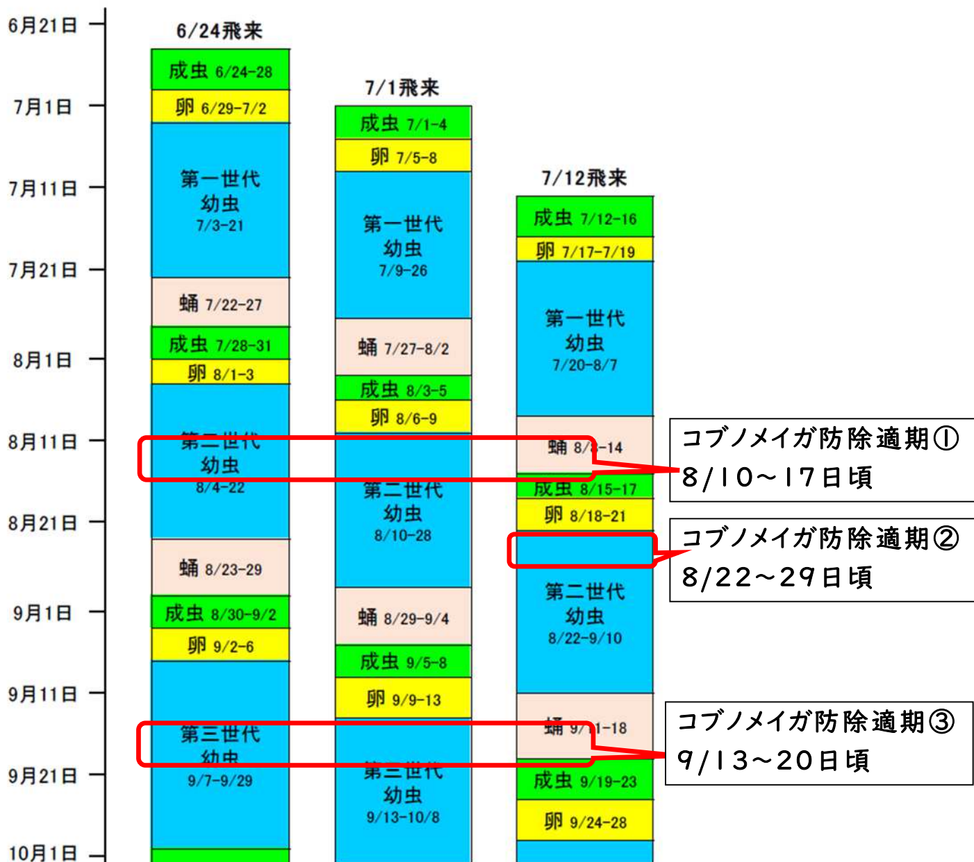
図2 コブノメイガ各世代の発生予測（第2版、2024年7月19日作成）
