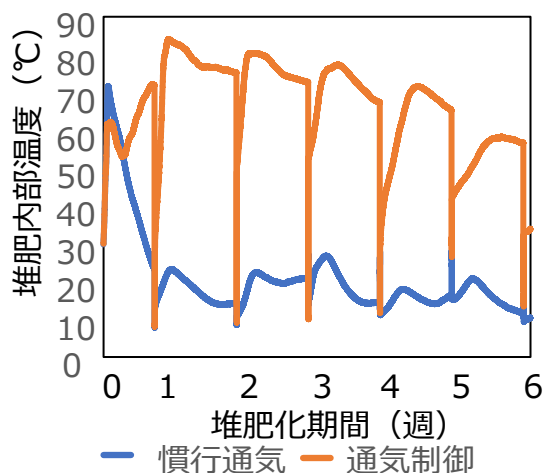
冬季の堆肥温度推移
