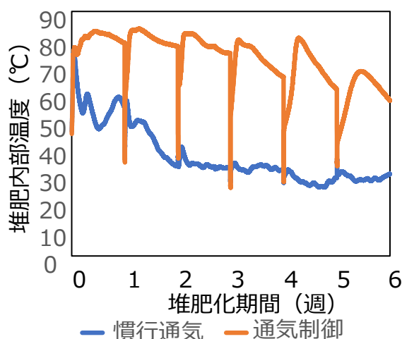
夏季の堆肥温度推移
