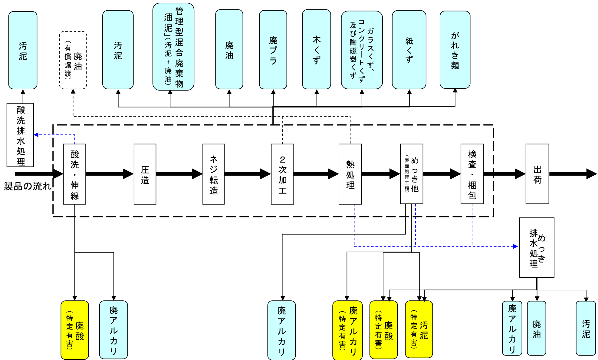
別紙 産業廃棄物の排出工程 (製造工程フロー図)
