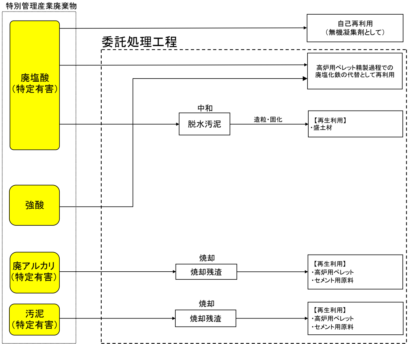
別紙 特別管理産業廃棄物の一連の処理の工程 (廃棄物処理フロー図)
