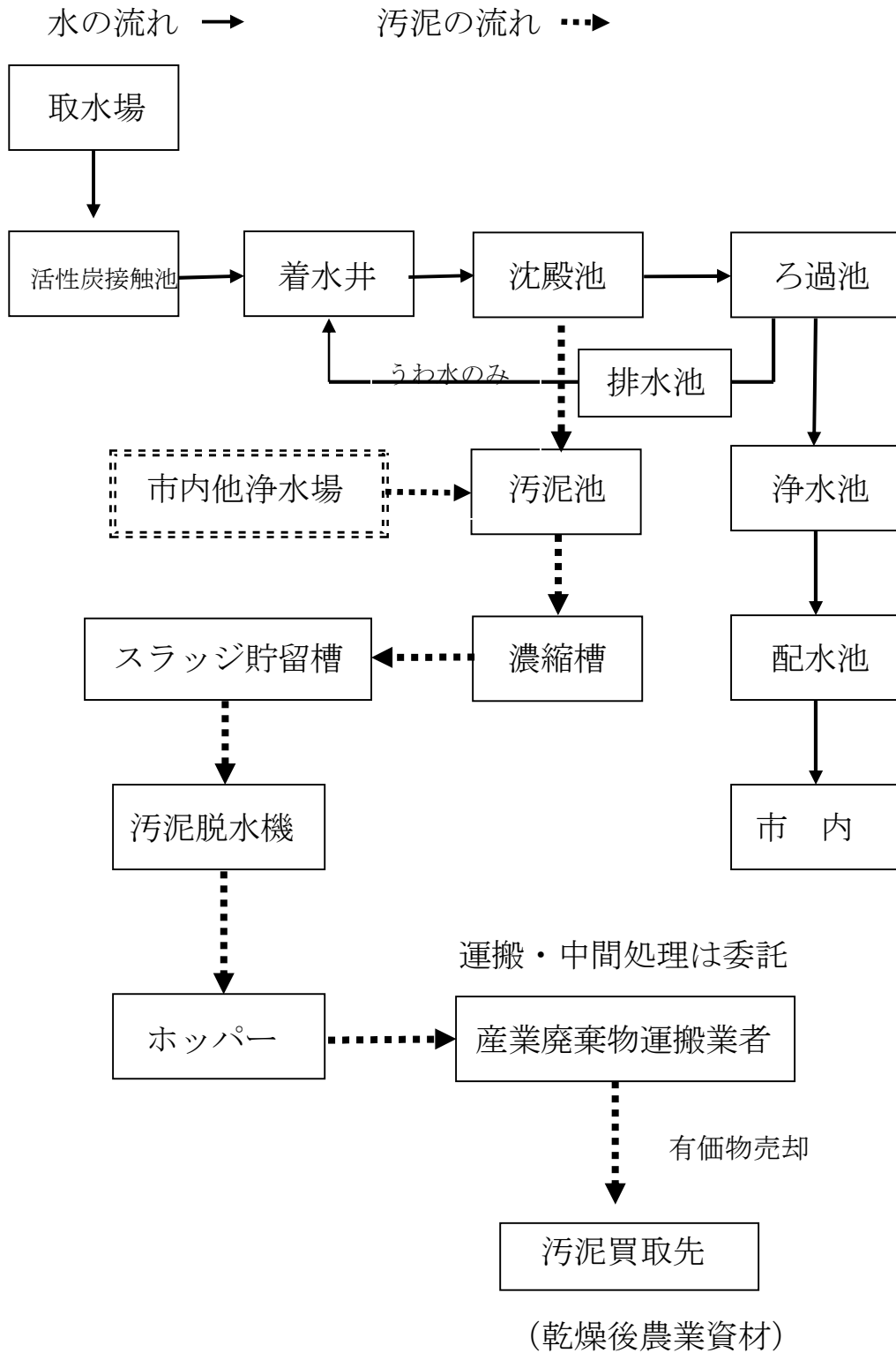
浄水場排水処理フロー図（久里浄水場）
