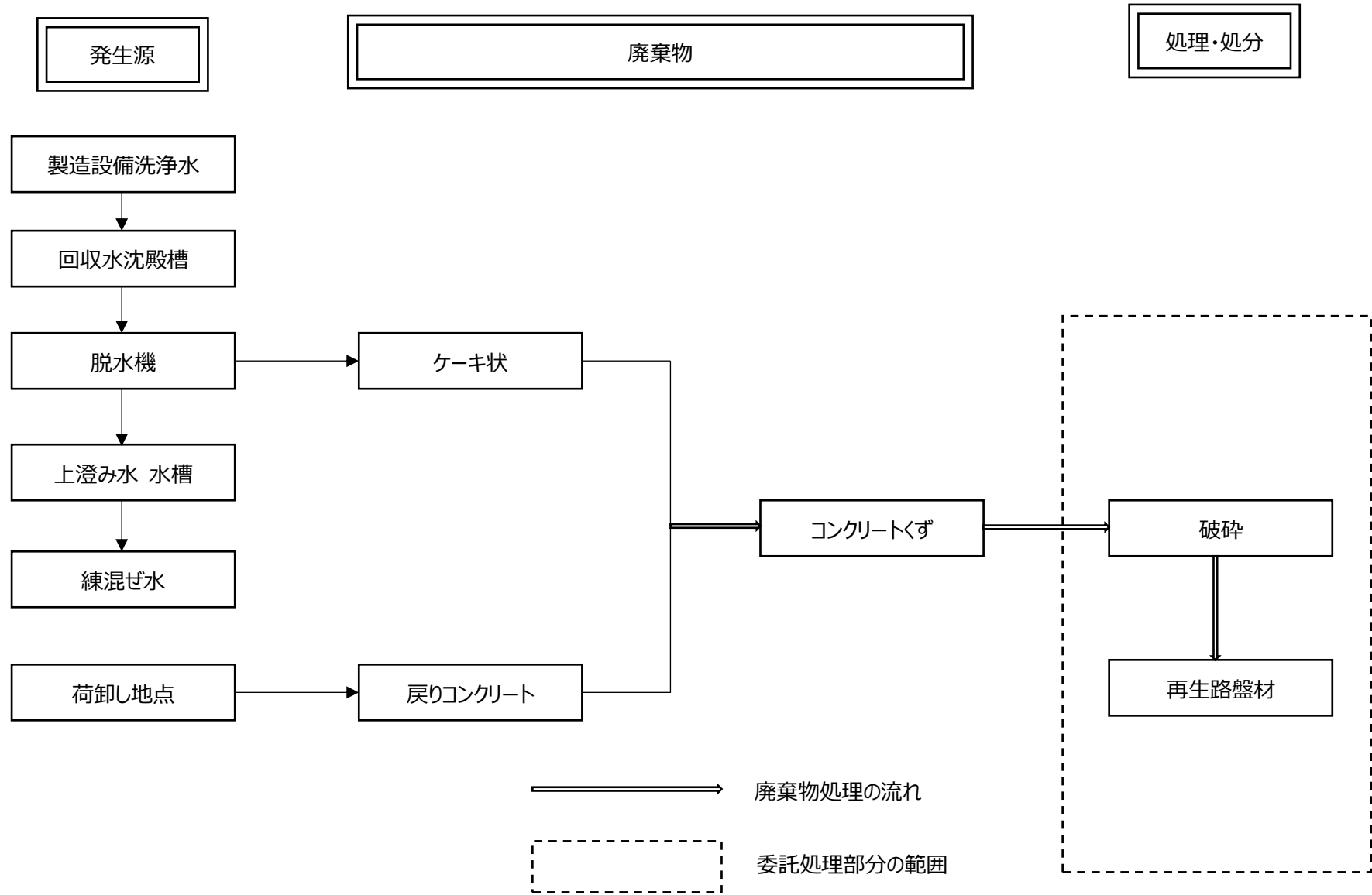
別紙①：④産業廃棄物の一連の処理工程
