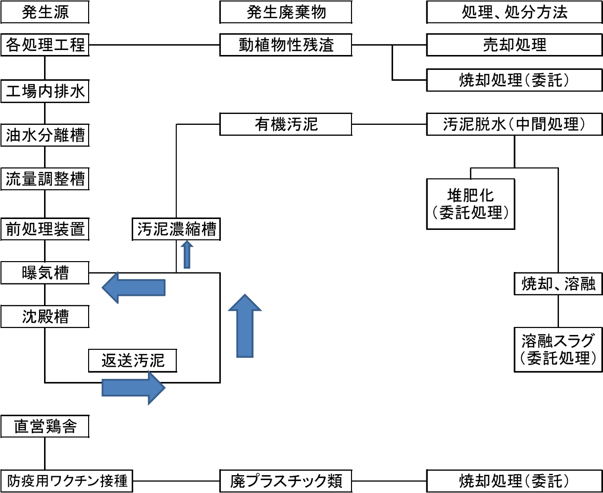
産業廃棄物処理フロー図
