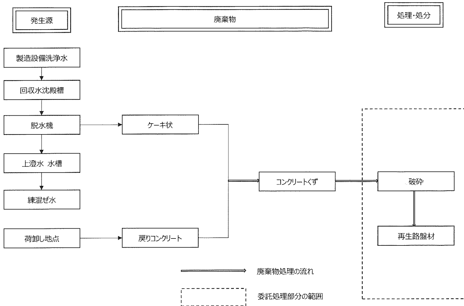
別紙①：④産業廃棄物の一連の処理工程
