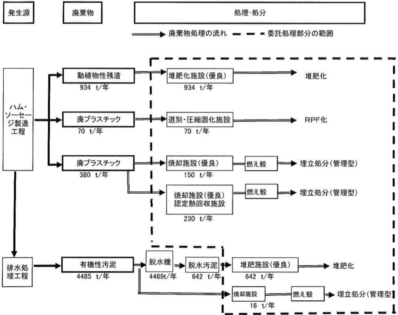
廃棄物処理フロー図(令和 5年度計画)
