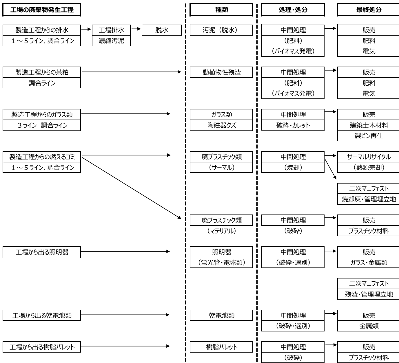
工場の廃棄物発生フロー図
