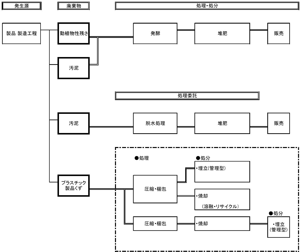
廃棄物処理の流れ
