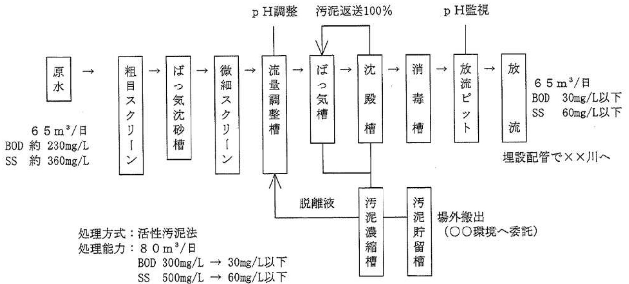
別図6 污水等の処理系統図 (例示)
