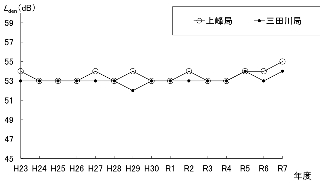
図1 通年局における L_{den} の経年推移
