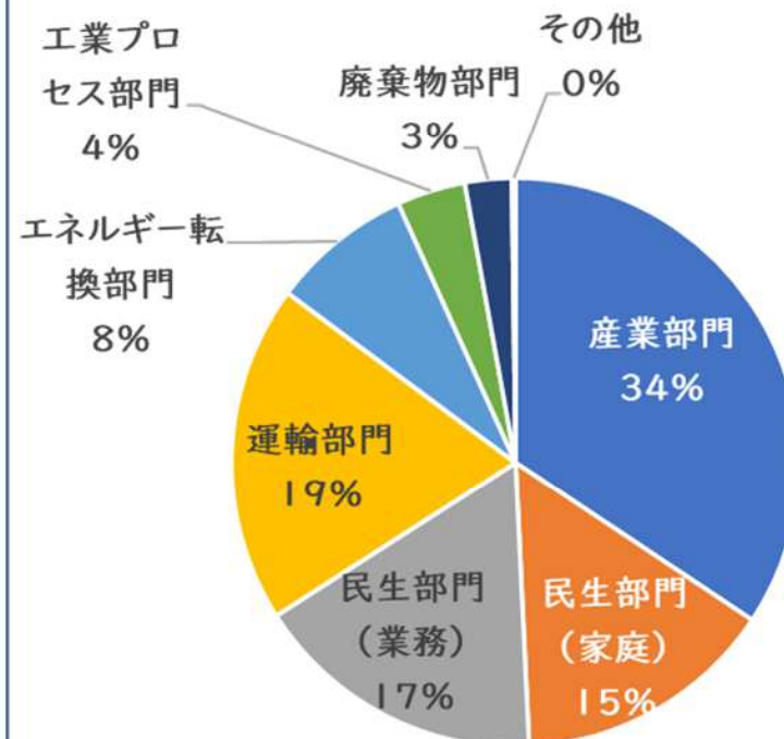
部門別排出量の構成【全国】(2023年度)
