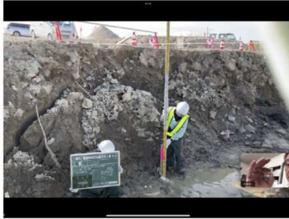
【立会状況（現場側）土工の出来形管理】
