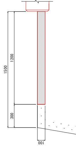
張コンクリート S=1:10
