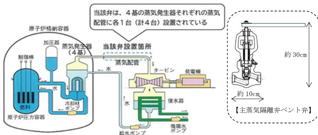
【発電所概要図】
