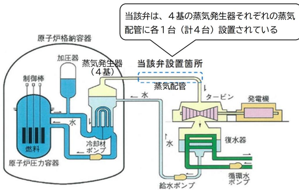
【発電所概要図】
