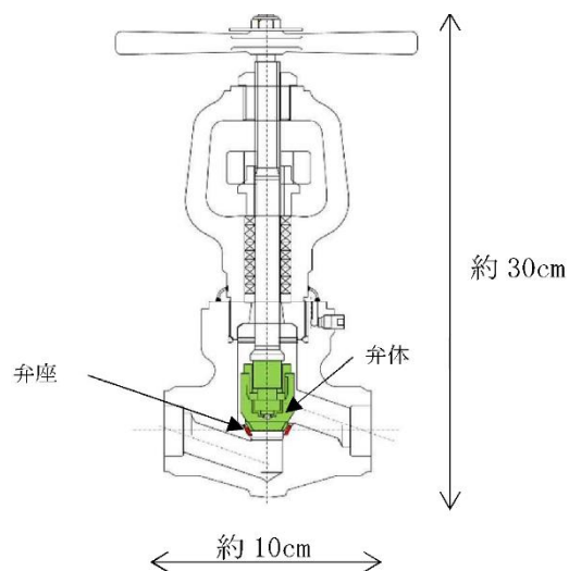
【蒸気配管設備の検査に使用する弁】
