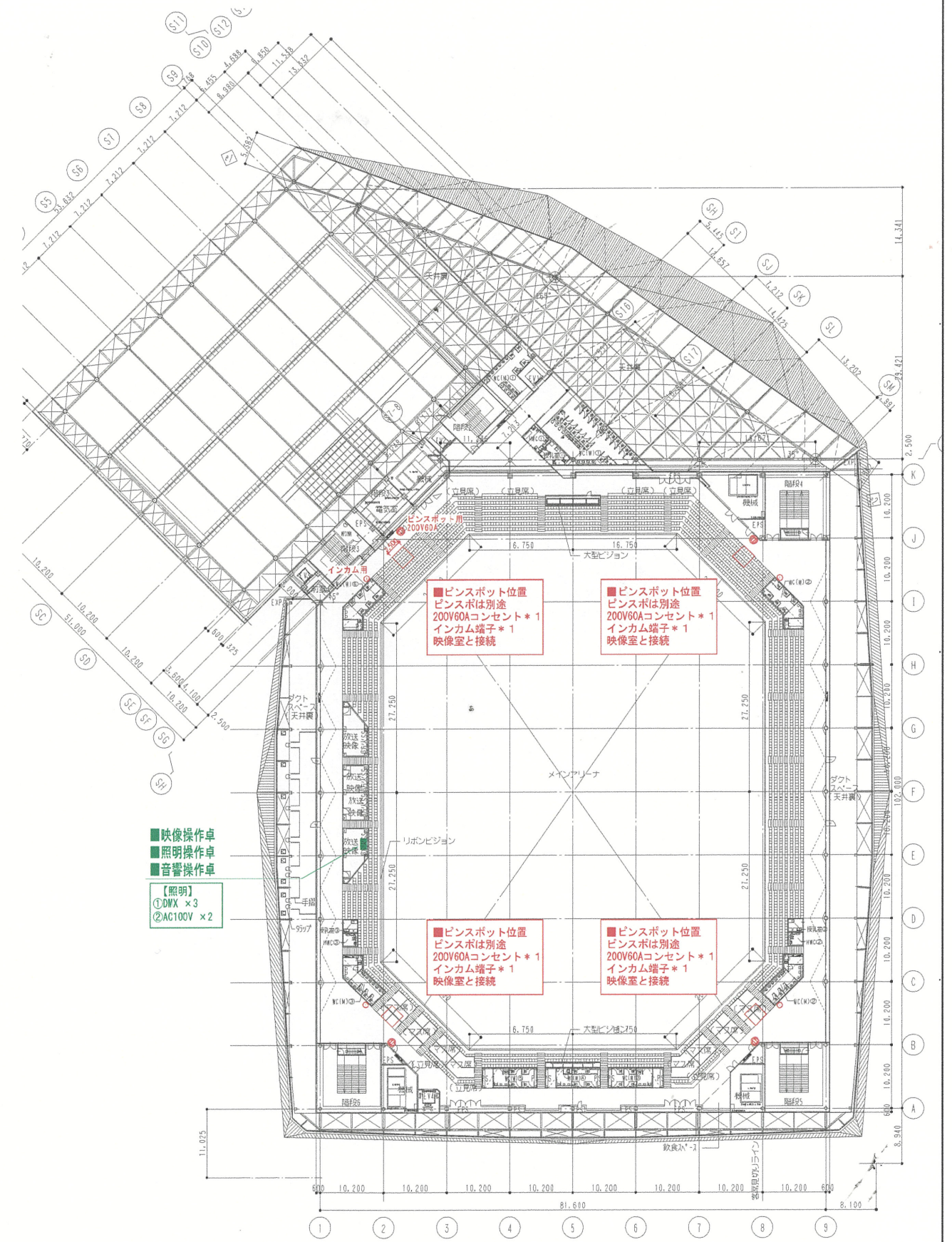
4階平面図
