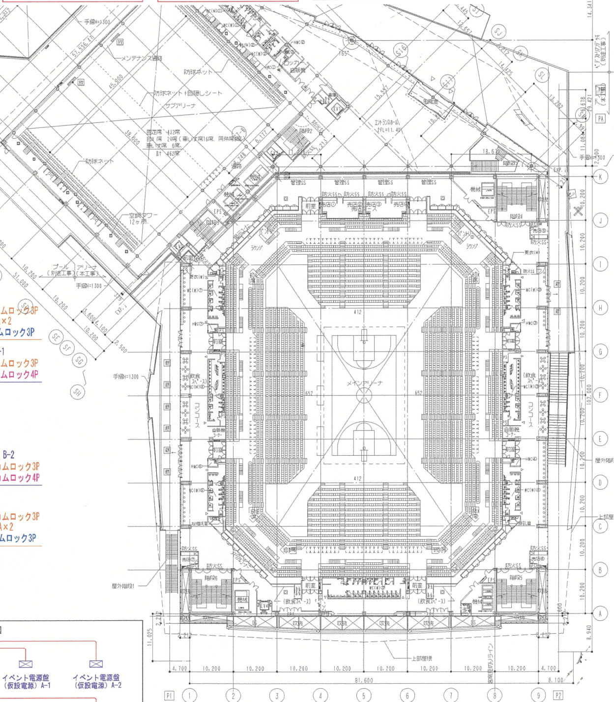
2階平面図
