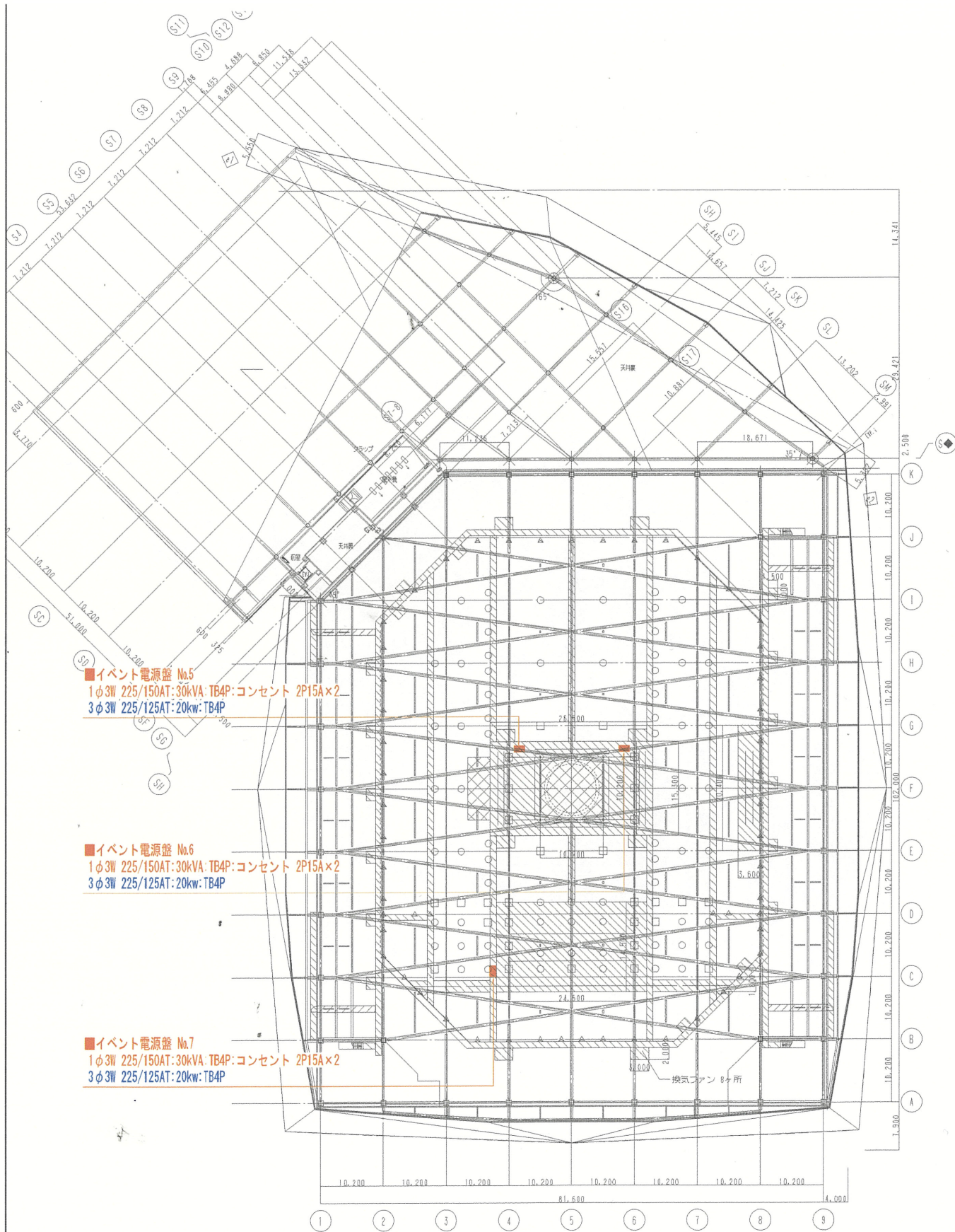
CW階平面図
