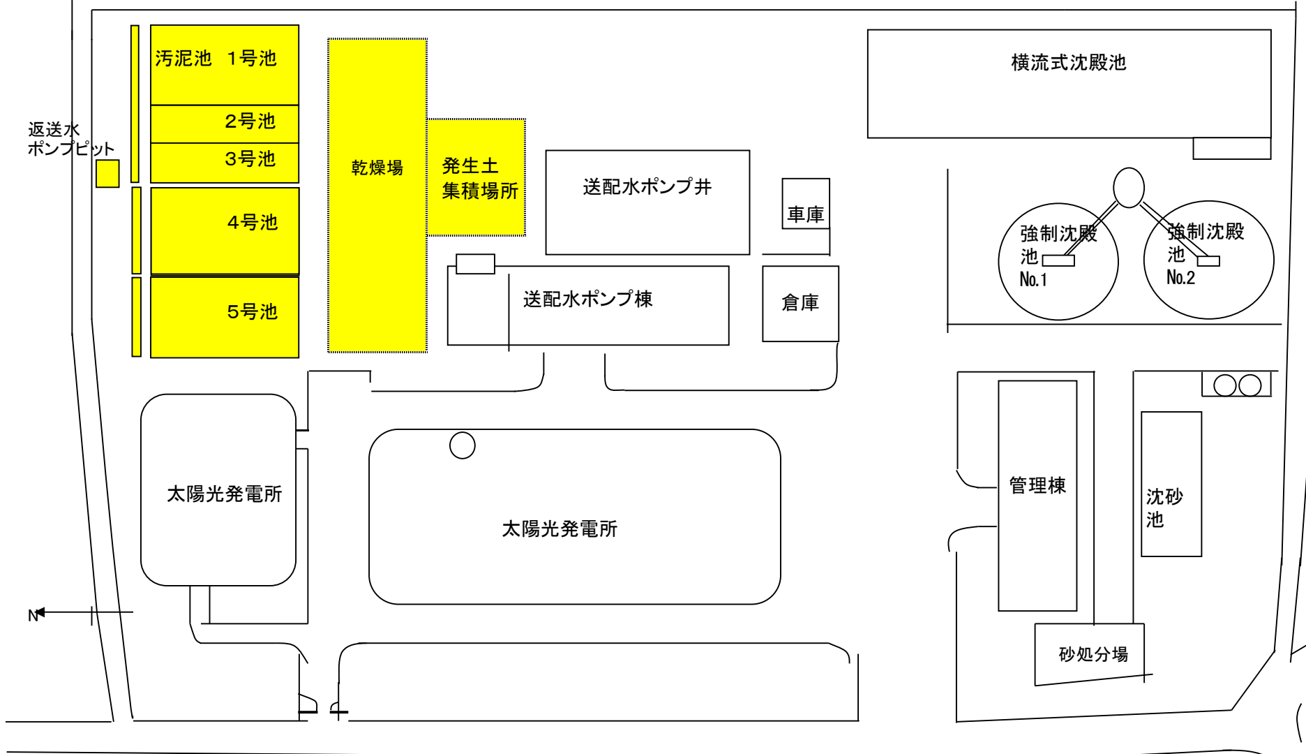
東部工業用水道浄水場配置(見取り)図
