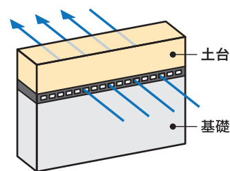
基礎パッキンによる床下換気
