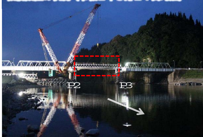
仮橋設置の状況 (令和2年8月21日時点)
