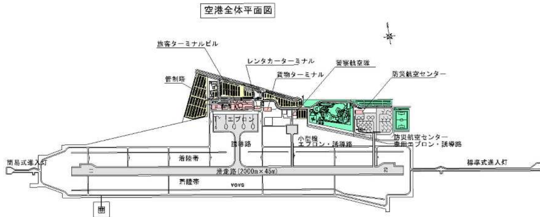
図 2.1-2 空港平面図
