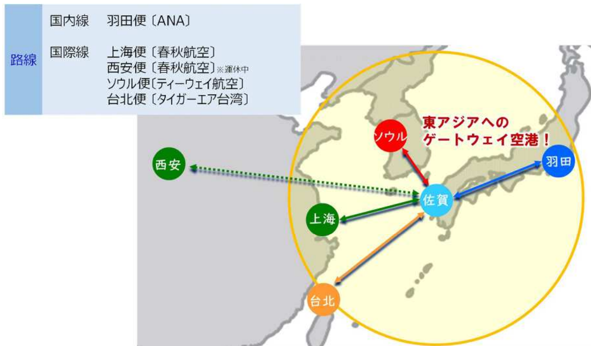
図 2.1-6 路線図
