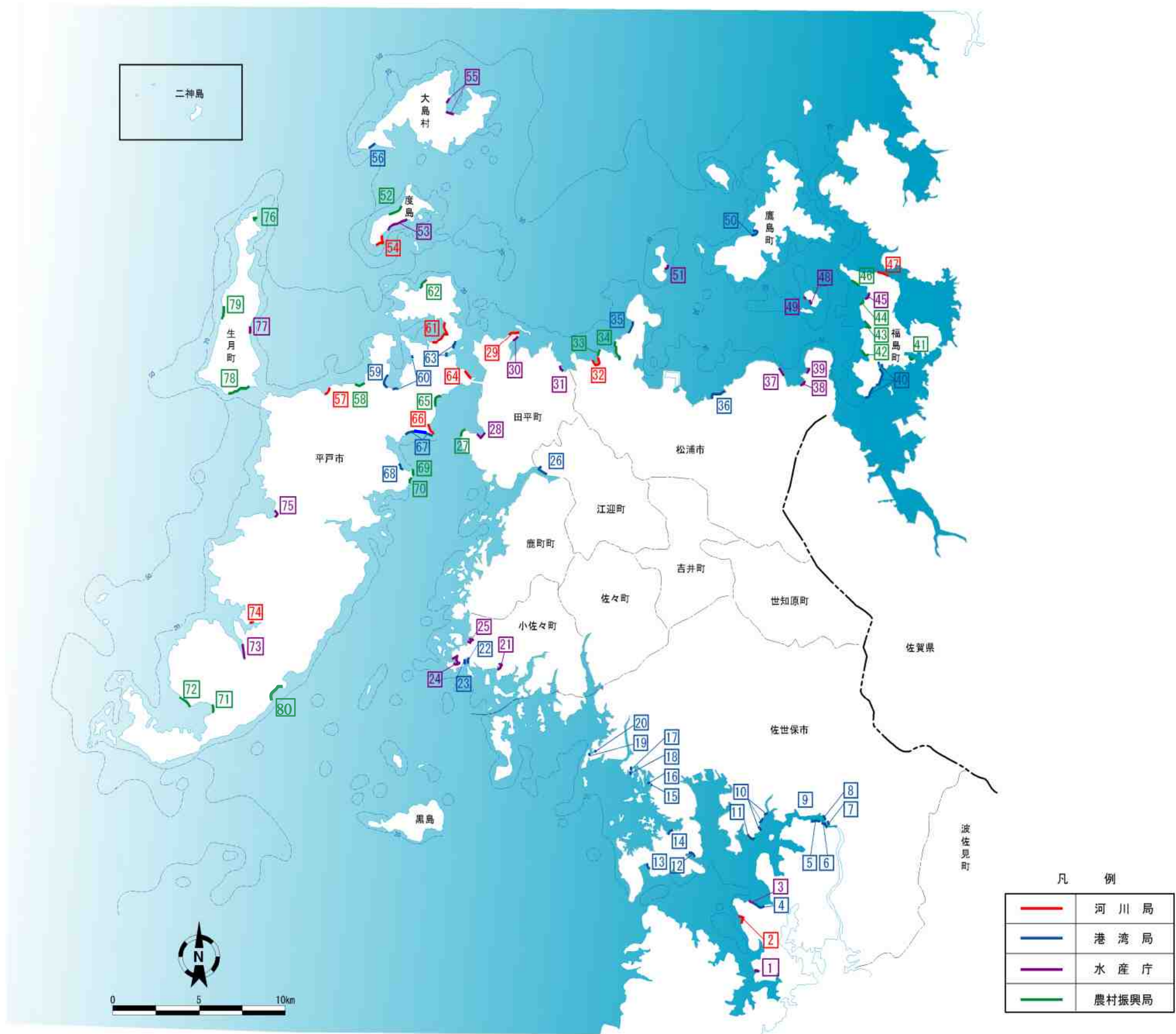
図 2.2 海岸保全施設を整備しようとする区域
