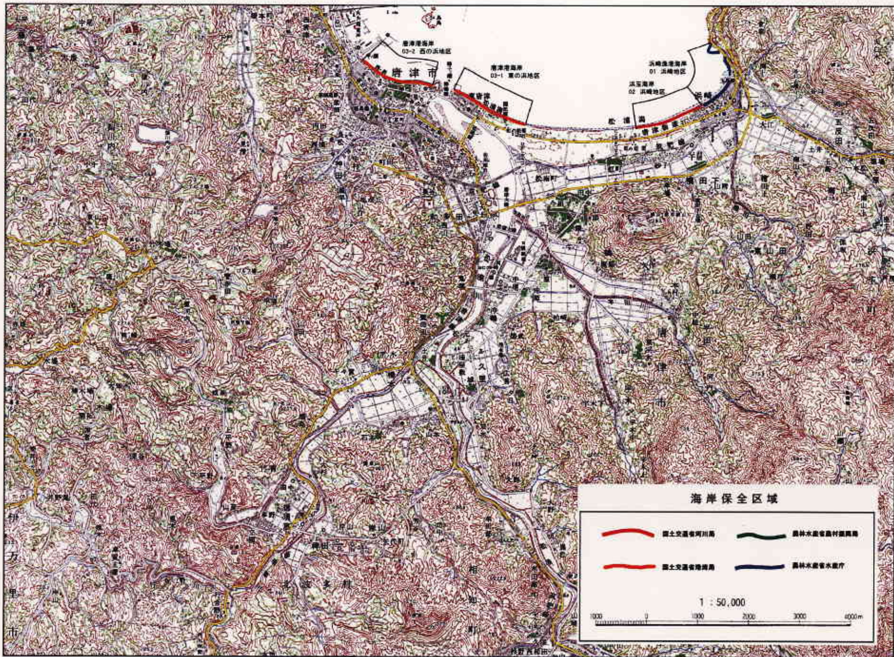
図2.1 海岸保全施設の配置
