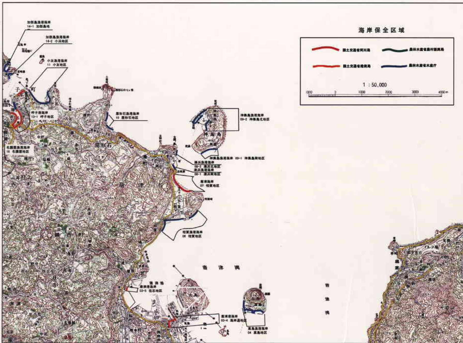
图2.1 海岸保全施設の配置
