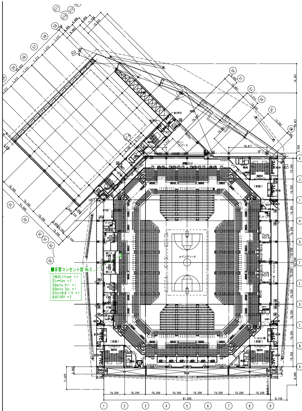
3階平面図
