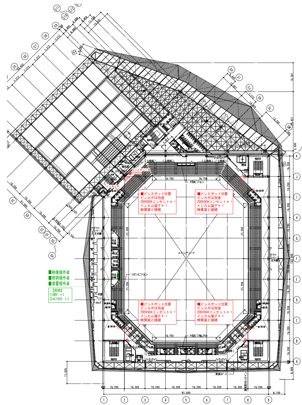
4階平面図
