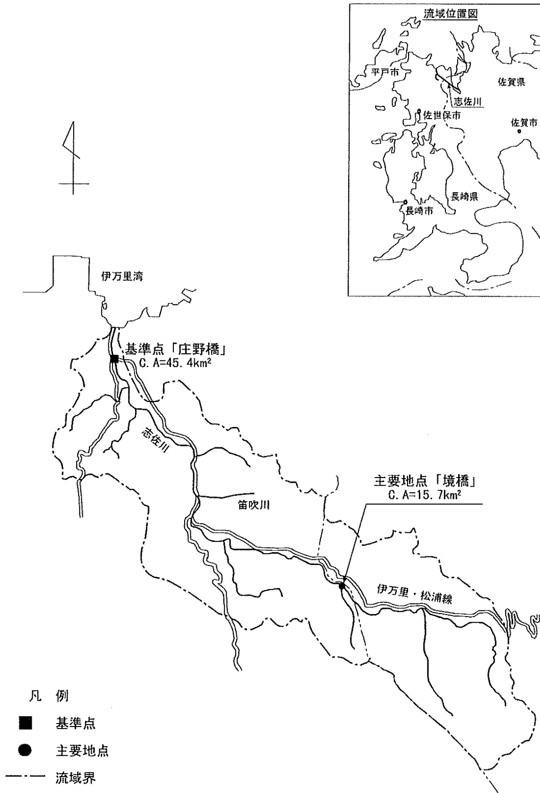
参考図 志佐川水系流域概要図(S=1:100,000)
